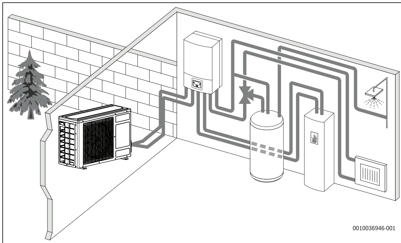
sl. 2 Toplotna pumpa za spoljnu jedinicu, AWS B unutrašnja jedinica bez električnog dogrevača, spoljni bojler za toplu vodu i spoljni pomoćni grejač
