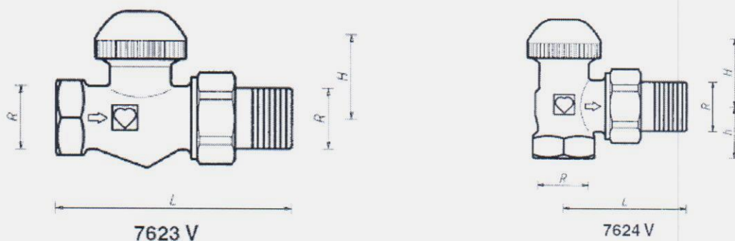
Slika 1. Izgled i dimenzije ventila HERZ-TS-98-V artikl br. 7623 V i 7624 V
